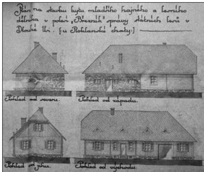
Plán na výstavbu domku lesního personálu a první strana stavebního deníku. (zdroj: Státní oblastní archiv Třeboň)
